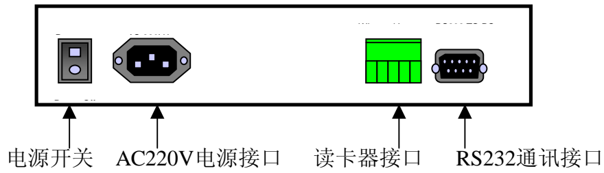
L-04后面板接口示意图
